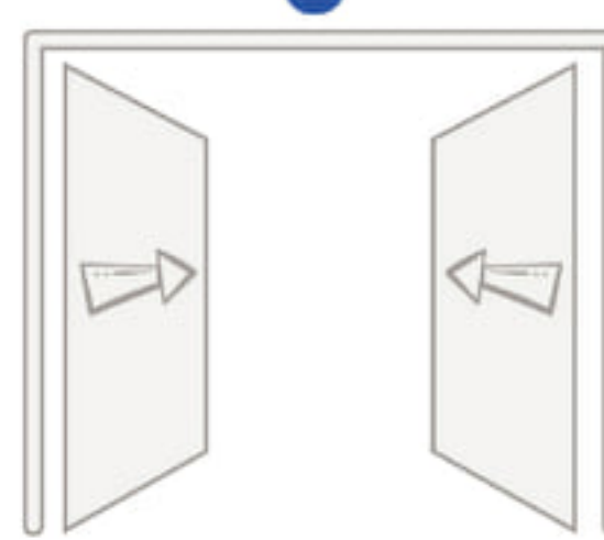
CMB2016
