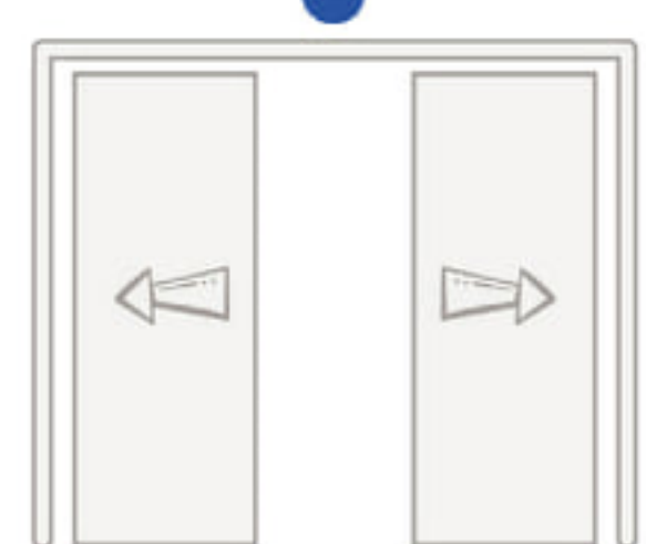
CMB2018
